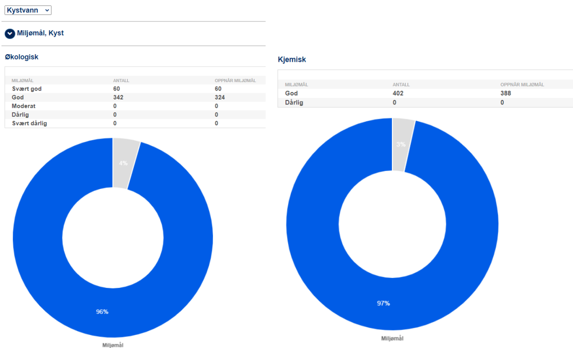
Figur 5-11. Miljømal for Kystvann i Troms og Finnmark vannregion. Kilde: vann-nett.no, 9/5-2023.
