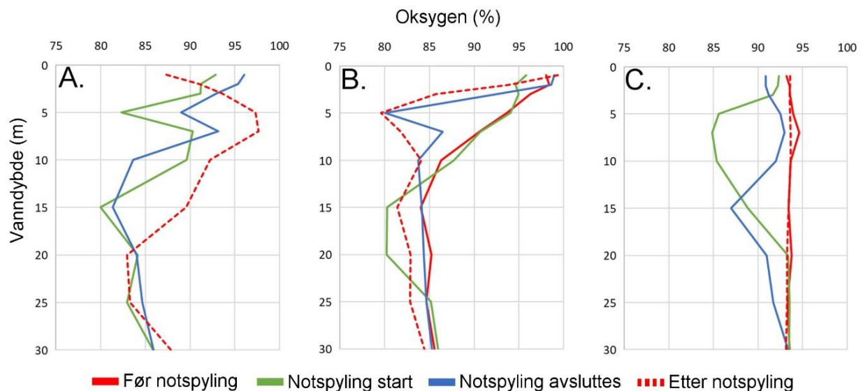
Figur 61. Profilmålinger av oksygen før, under og etter notspyling. Oksygennivåer oppgitt som metning (%).
