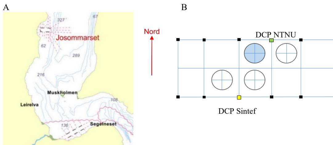
Figur 11. A viser plassering av anlegget på Josommarset og B viser anleggsconfigurasjonen med de aktive merdene med markering av ADCP- og DCP-plasseringene. Merd i blått er forsøksmerden.
