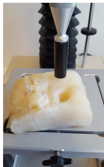
Bilde 5 Teksturanalyse av klippfisk med bruk av flat sylinderprobe
