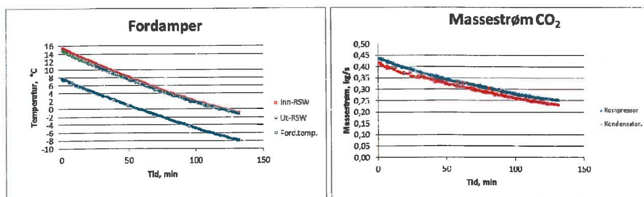
Figur 3. Test 1. Målt RSW- og fordampningstemperatur samt CO 2 -massestrøm under RSW- nedkjøling.
