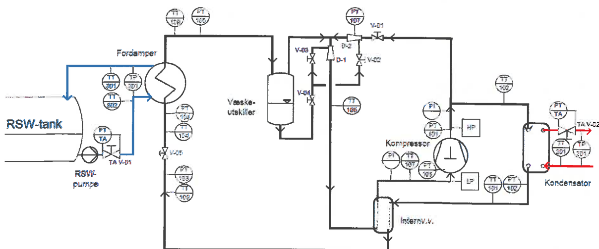
Figur 1. Prosess- og instrumentering. Forkortelse TT for temperatur, TP for temperaturdifferanse, PT for trykk og FT for volumstrøm.
