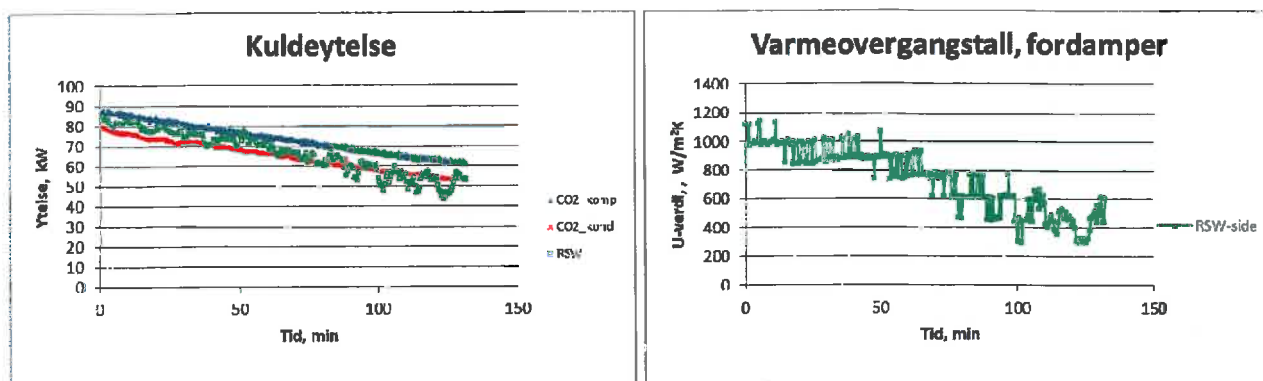
Figur 2. Test 1. Målt kuldeytelse og varmeovergangstall i fordampere under RSW- nedkjøling.
