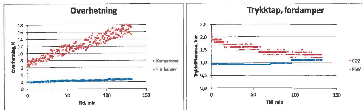
Figur 4. Test 1. Målt overhetning ut av fordampere og inn på kompressor samt fordampetrykktap på CO 2 og RSW-side under RSW- nedkjøling.
