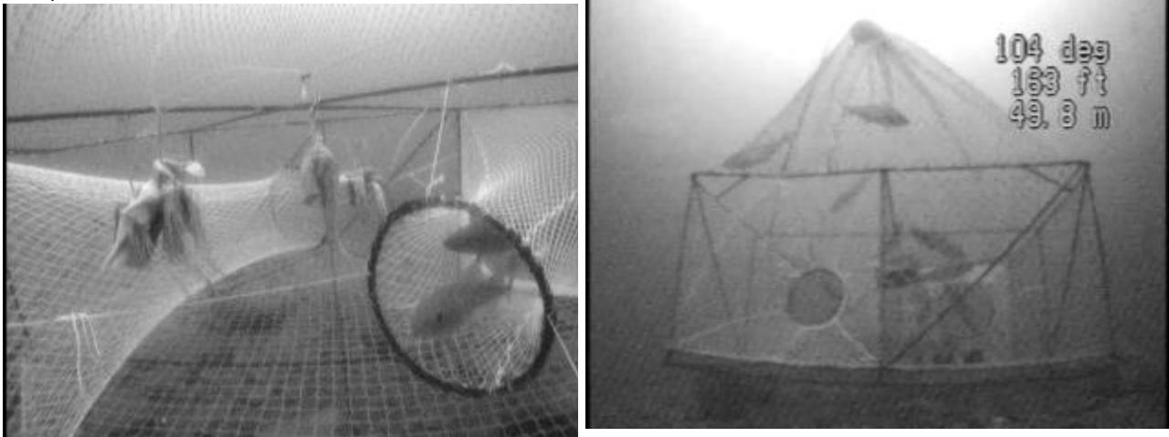
Bilde 4 Undervannsoptak av teine fra Newfoundland, vi ser fisk som går inn og fisk som trekker opp i den flytende takkonstruksjonen.
