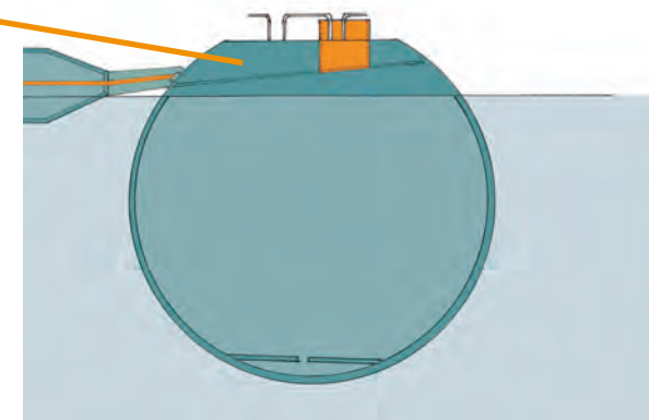
Fôrsilo koblet til energi og forslange sett fra siden.
