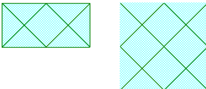
Figur 3-5: Not 3. Not med skrå tau og diamond-orientert notlin (side til venstre og bunn til høyre). 12 meter dyp.
