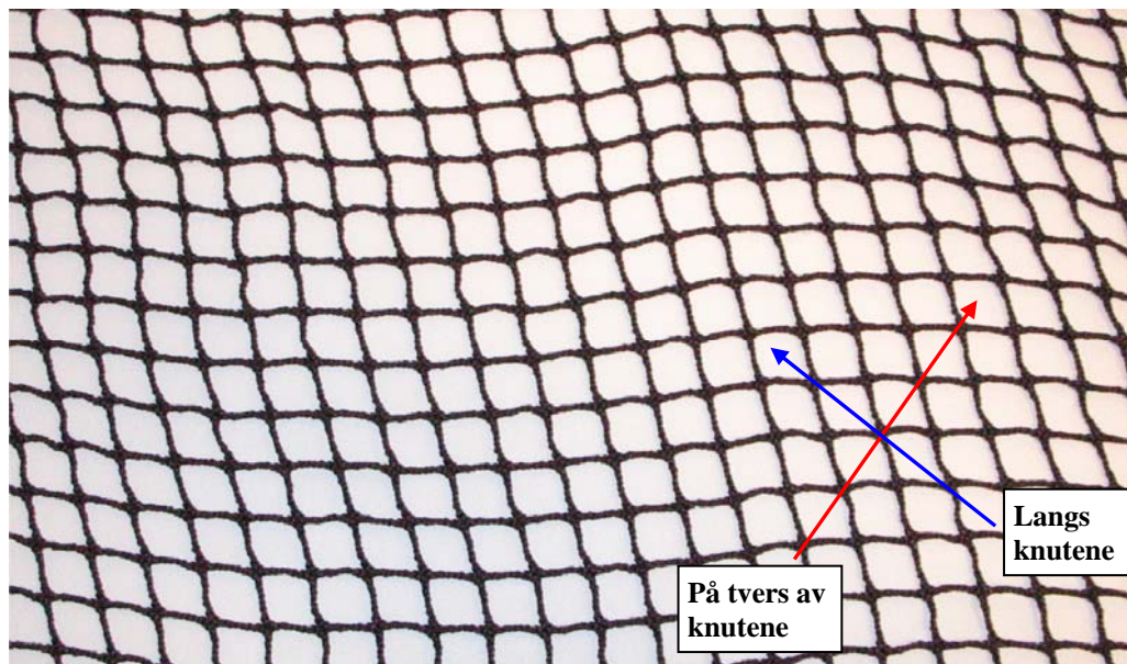
Figur 3-10: Flaggorientert notlin. Notlinet vil ha forskjellig stivhet i de to retningene diagonalt på maskene. Disse retningene er kalt ”på tvers av knutene” og ”langs knutene”.
