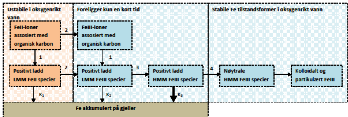
Figur 3 Skjematisk modell for transformasjon av tilstandsformer av Fe i ustabile driftvannsblandsoner. FeII er kilden til FeIII avsetningen på gjeller til fisk. LMM står for "Lavmolekylært" og HMM står for "Høymolekylært". Reaksjonshastighet avtar K_3 > K_2 > K_1 .
