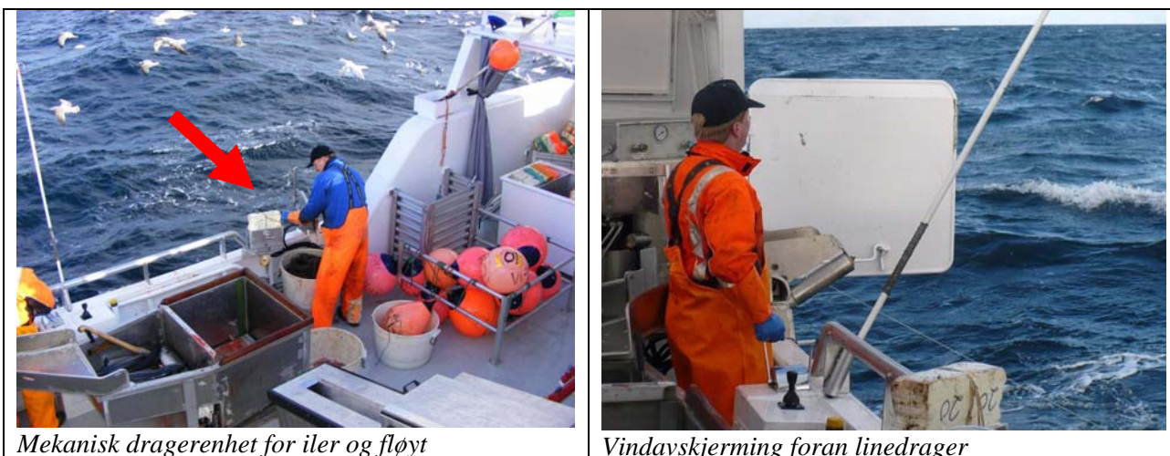
Bilde 12 Operatører ved ilehaler (venstre) og under draging med vindskjerm (høyre)
